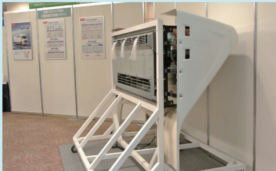
デンソーの車載用冷凍装置
